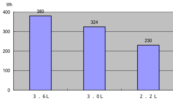
サイズ別の沸騰1回あたりの消費電力量(グラフ4)
